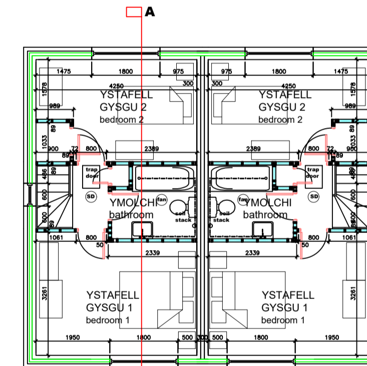
CYNLLUN Y LLAWR CYNTAF first floor plan
