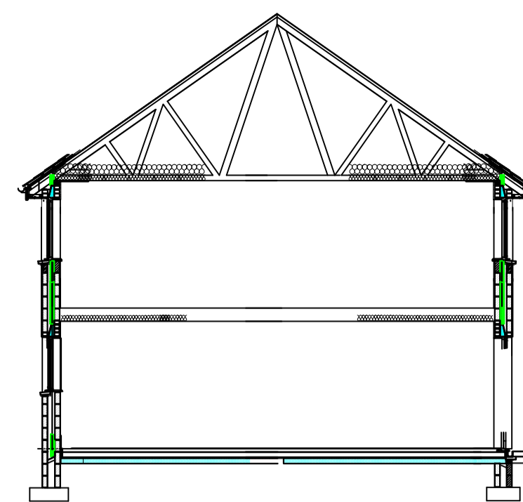
TORIAD A-A section A-A
