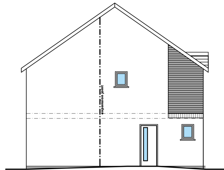
EDRYCHIAD OCHR side elevation
