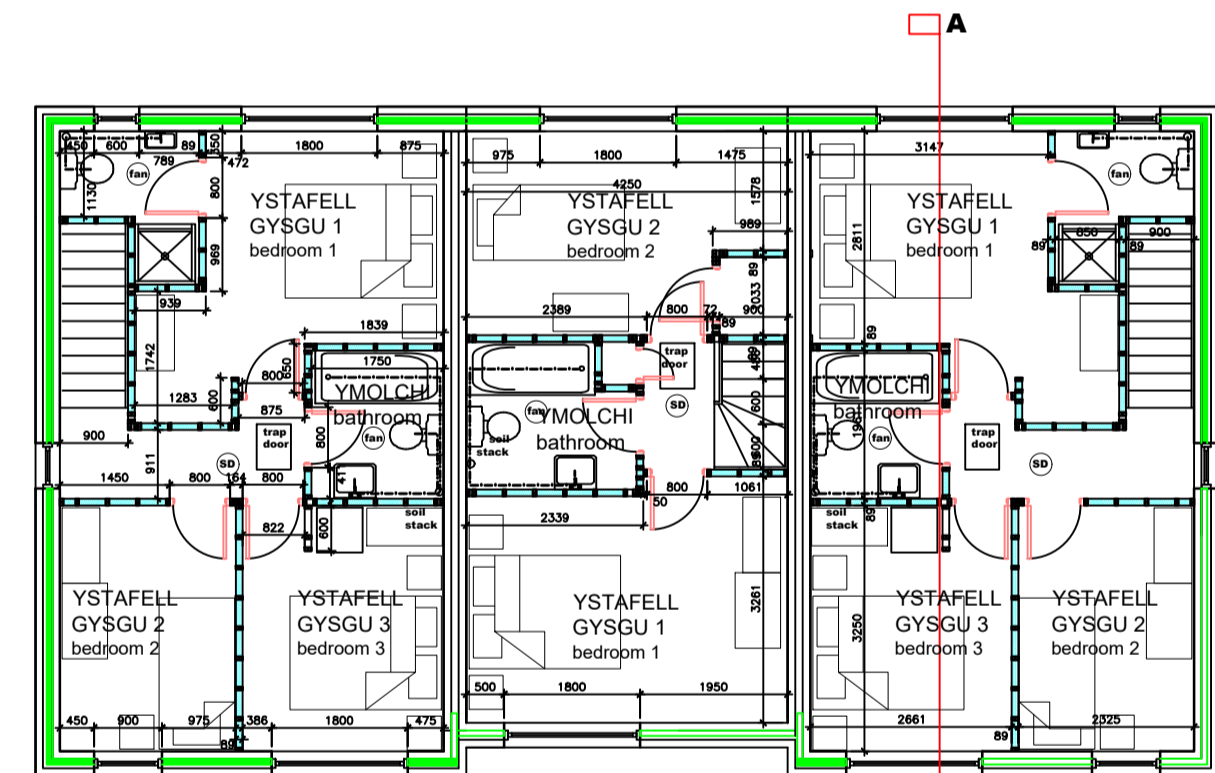
CYNLLUN Y LLAWR CYNTAF first floor plan
