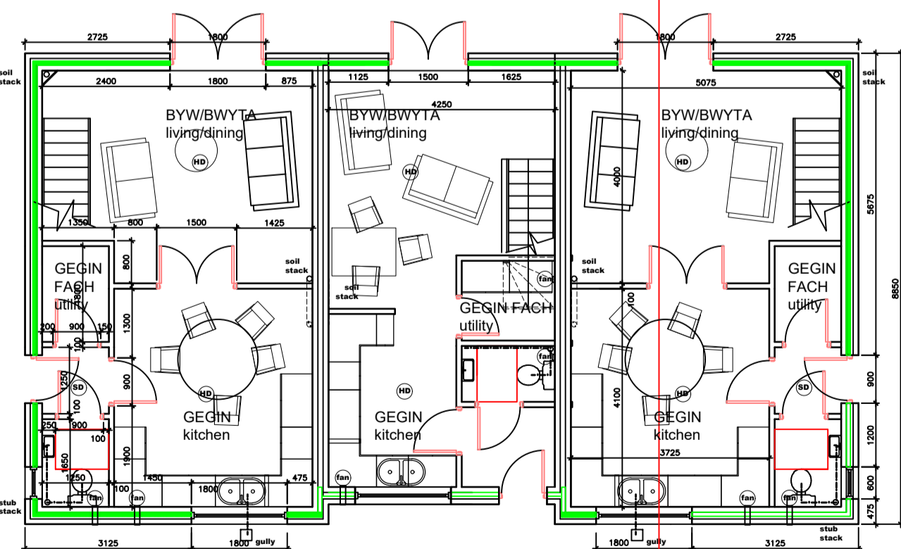
CYNLLUN Y LLAWR GWAELOD ground floor plan
