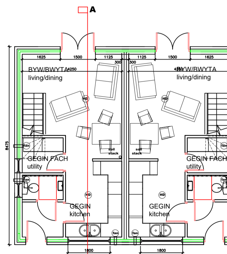
CYNLLUN Y LLAWR GWAELOD ground floor plan
